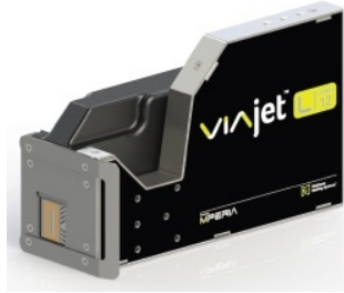
VIAjet L-Series - tlačová hlava L12
